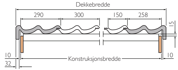
Bruk av gavlstein for Zanda betongtakstein.
